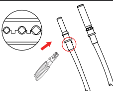
Rys. 5.4 Zaciśnij pin kontaktowe do przewodu
