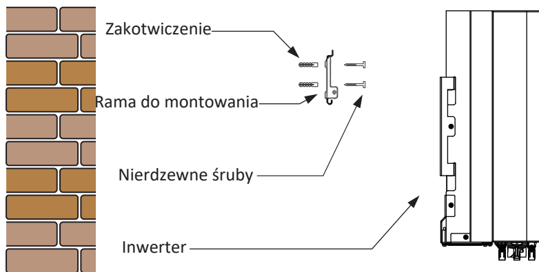
Rys. 4.4 Instalacja Inwertera
