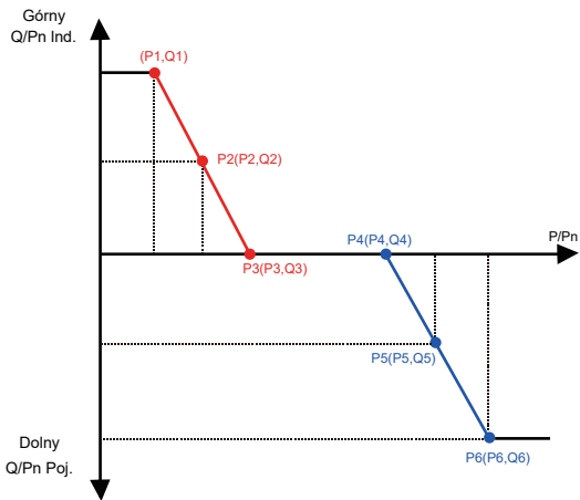
Rys. 8.31 Krzywa regulacji mocy biernej w trybie Q(P)
