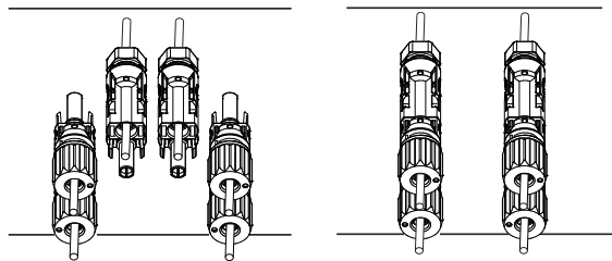
Rys. 5.6 Połączenie wejścia DC
