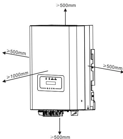
Rys. 4.3 Przerwa Instalacyjna
