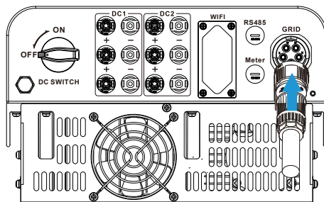
Rys. 5.10 Połączenie wejścia AC
