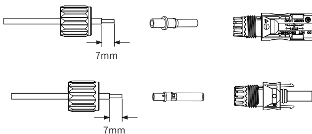
Rys. 5.3 Zdejmowanie nakrętki złącza
