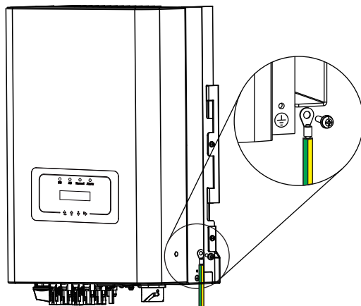
Rys. 5.11 Instalacja obudowanego przewodu uziemiającego
