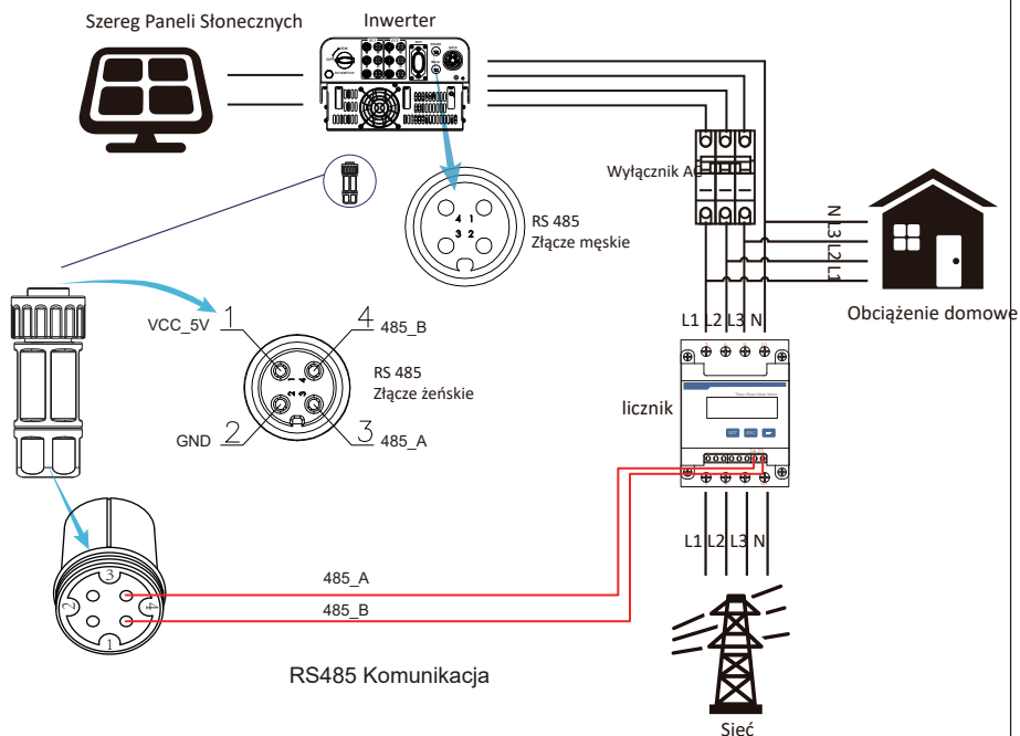
Rys 7.6 Schemat połączenia licznika CHNT
